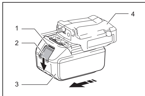
► 1. Voyant rouge 2. Bouton 3. Batterie 4. Porte-batterie (accessoire en option)
